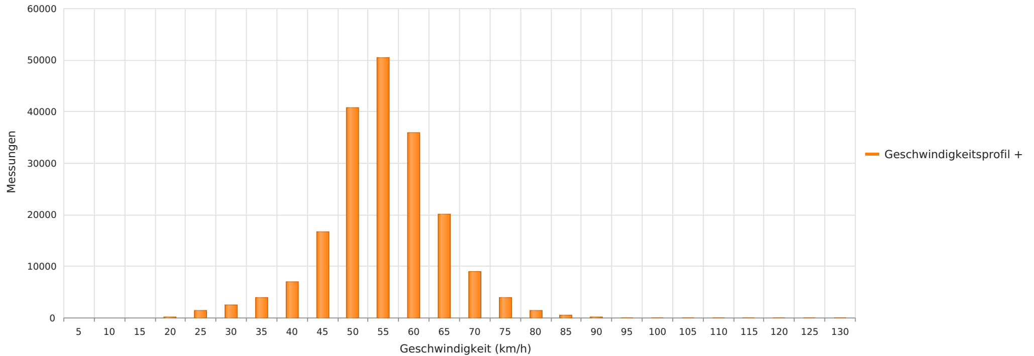
2023_07_28-08_29 Norddrebber Ortsausgang Richtung Gilten Anzahl der Messwerte vs. Geschwindigkeit
