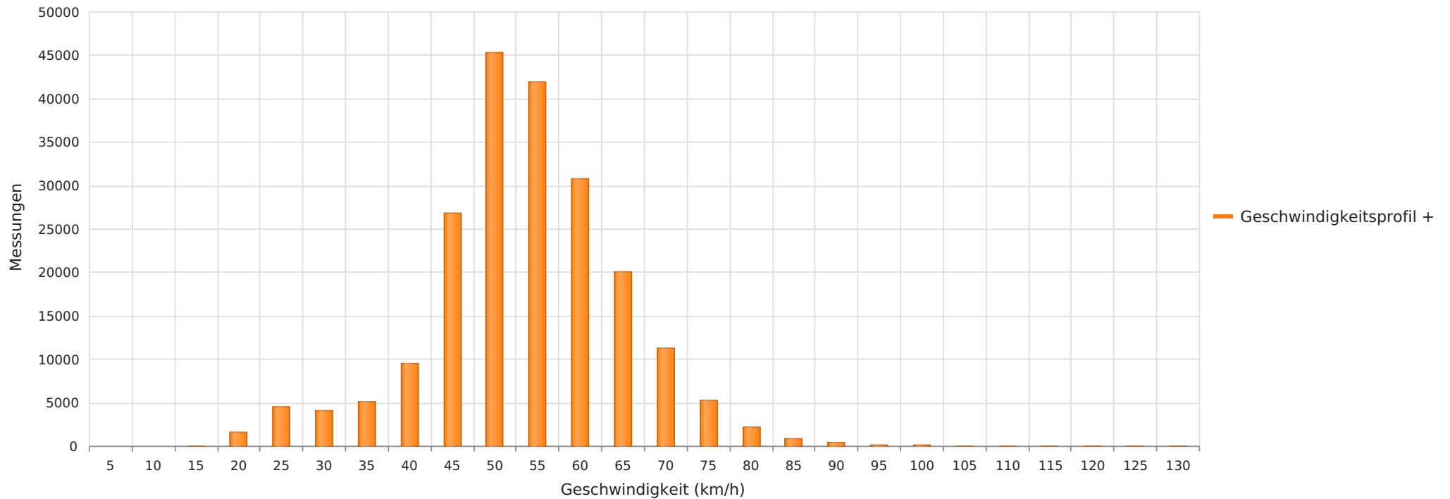
2023_11_01-12_07 Essel K105 Richtung Ortskern Anzahl der Messwerte vs. Geschwindigkeit
