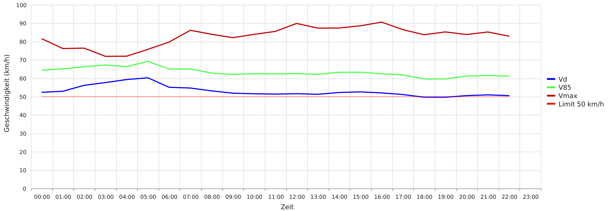
2023_11_01-12_07 Essel K105 Richtung Ortskern Vd, V85, Vmax vs. Uhrzeit
