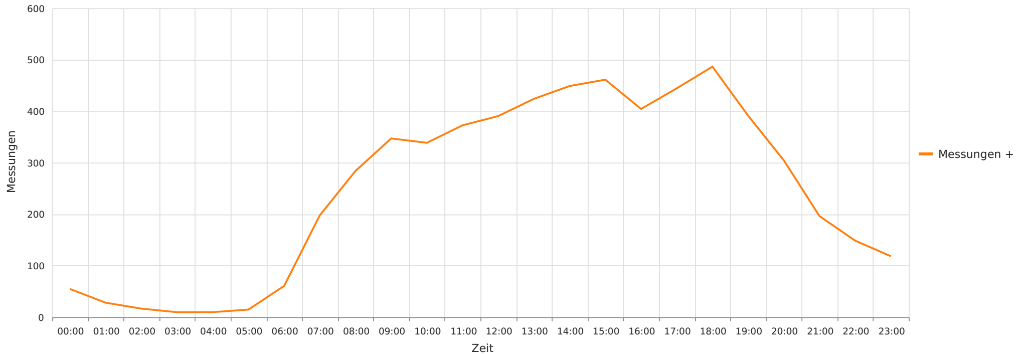
2023_11_01-12_07 Essel K105 Richtung Ortskern Gemittelte Anzahl an Messwerten vs. Uhrzeit
