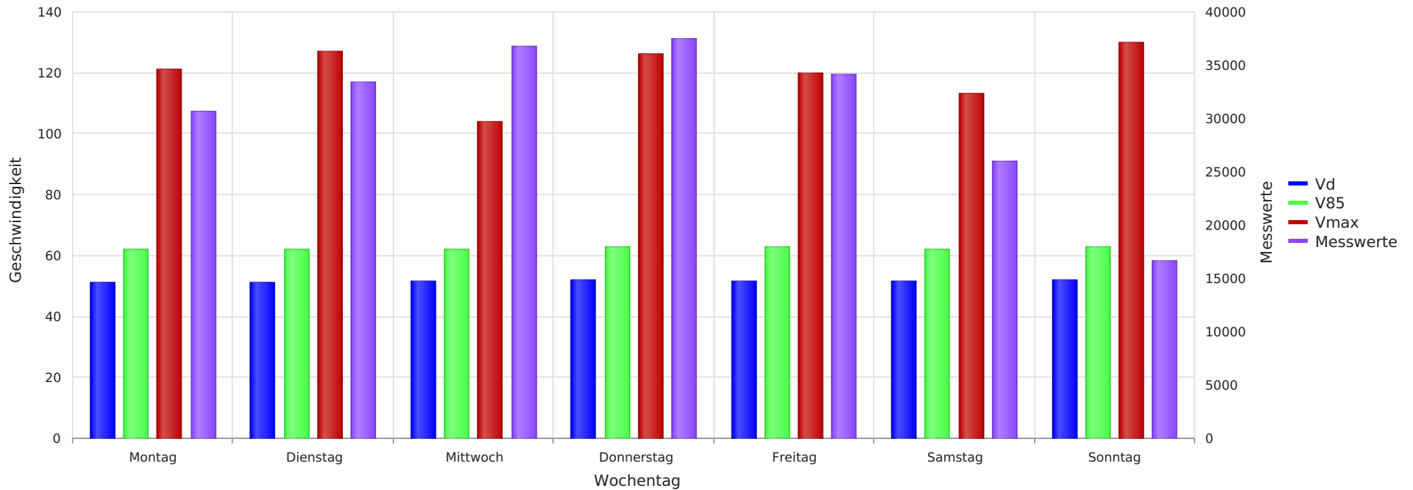
2023_11_01-12_07 Essel K105 Richtung Ortskern Vd, V85, Vmax, Anzahl der Messwerte vs. Wochentag
