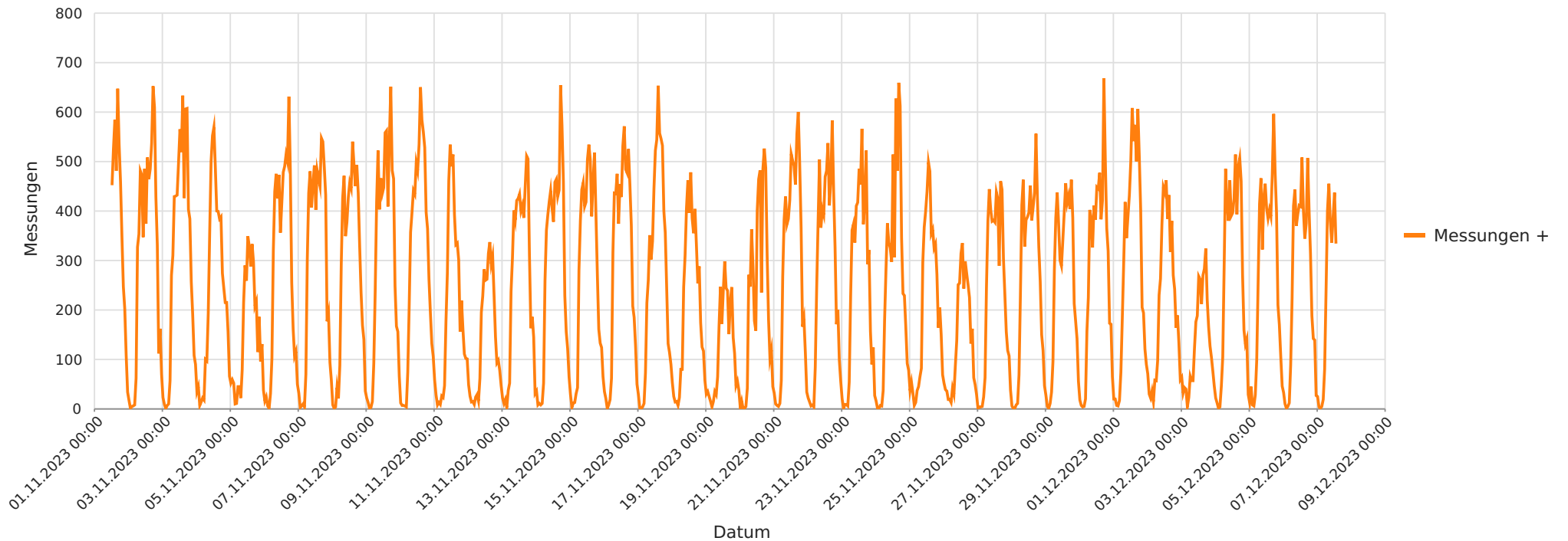
2023_11_01-12_07 Essel K105 Richtung Ortskern Anzahl der Messwerte vs. Messzeitraum
