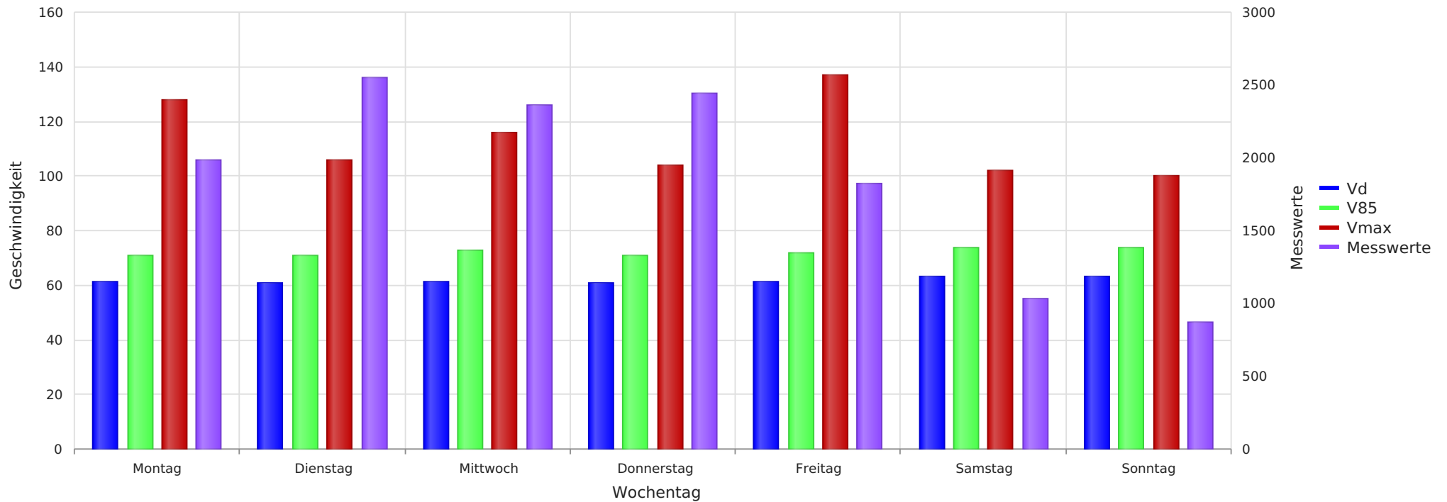
2023_12_11-12_22 Engehausen Ortseingang Richtung Winsen Vd, V85, Vmax, Anzahl der Messwerte vs. Wochentag
