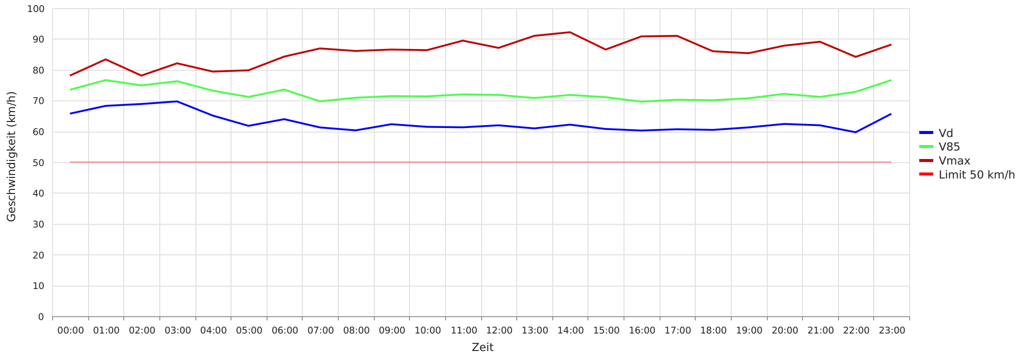
2023_12_11-12_22 Engehausen Ortseingang Richtung Winsen Vd, V85, Vmax vs. Uhrzeit
