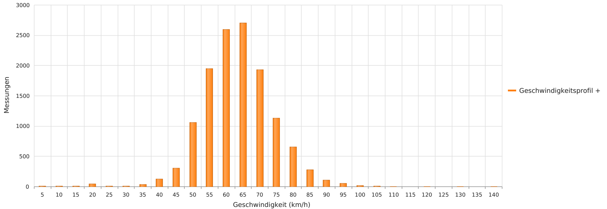
2023_12_11-12_22 Engehausen Ortseingang Richtung Winsen Anzahl der Messwerte vs. Geschwindigkeit
