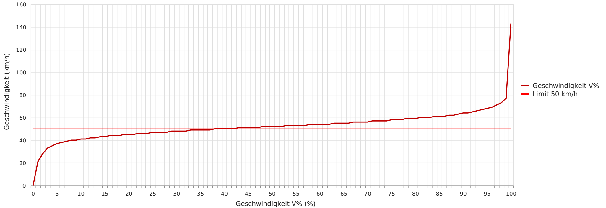
2023_12_15-2024_01_04 Buchholz B214 Richtung Celle Geschwindigkeit vs. prozentueller Anteil an Messwerten
