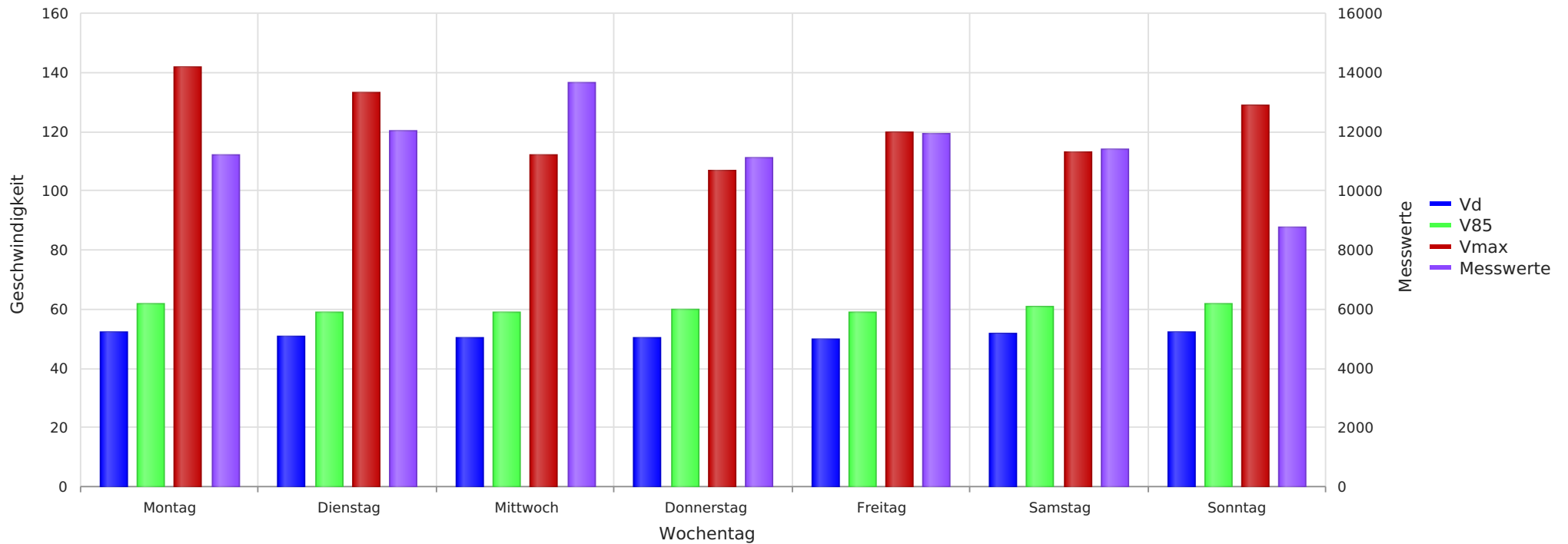
2023_12_15-2024_01_04 Buchholz B214 Richtung Celle Vd, V85, Vmax, Anzahl der Messwerte vs. Wochentag
