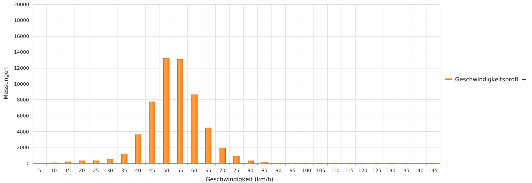
2023_12_15-2024_01_04 Buchholz B214 Richtung Celle Anzahl der Messwerte vs. Geschwindigkeit
