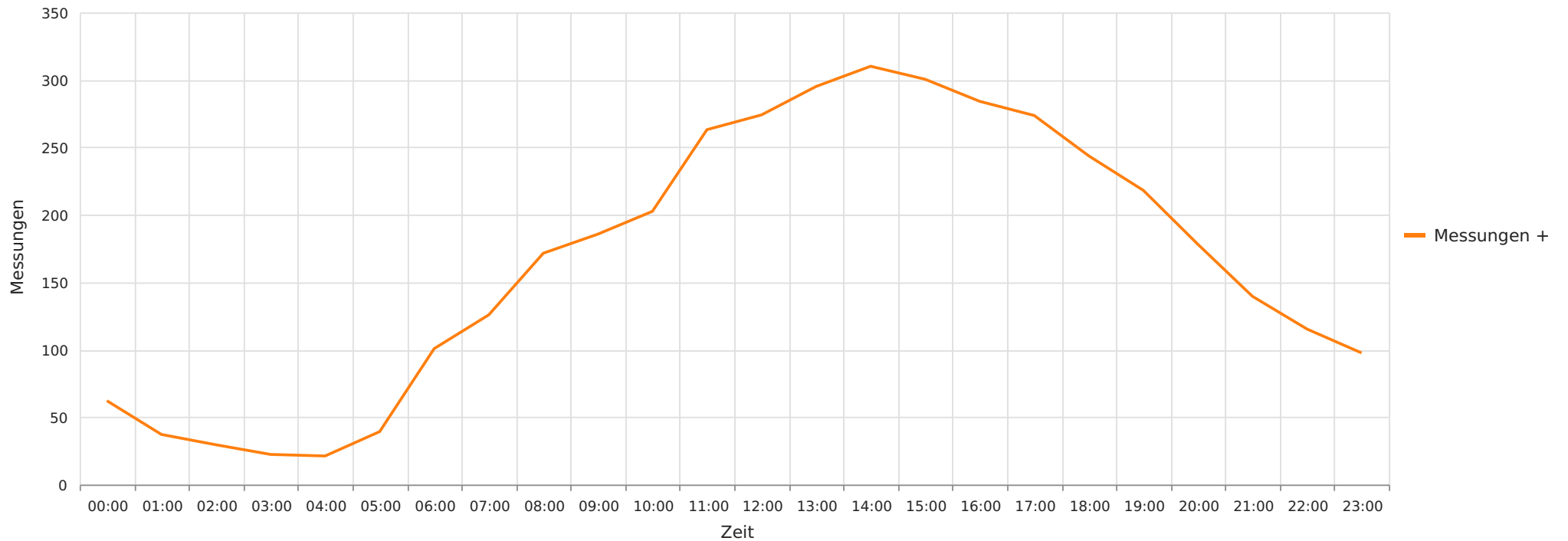
2023_12_15-2024_01_04 Buchholz B214 Richtung Celle Gemittelte Anzahl an Messwerten vs. Uhrzeit
