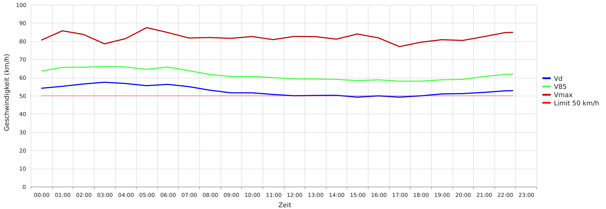
2023_12_15-2024_01_04 Buchholz B214 Richtung Celle Vd, V85, Vmax vs. Uhrzeit
