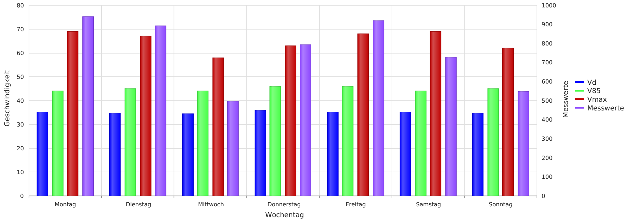
2024_01_11-01_24 Hope Am Schacht Richtung Adolfglück Vd, V85, Vmax, Anzahl der Messwerte vs. Wochentag
