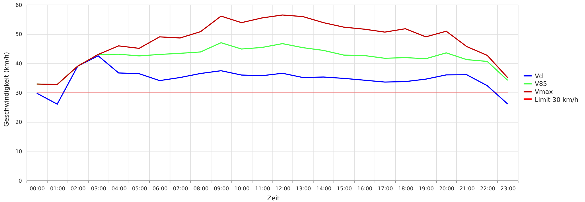
2024_01_11-01_24 Hope Am Schacht Richtung Adolfsglück Vd, V85, Vmax vs. Uhrzeit
