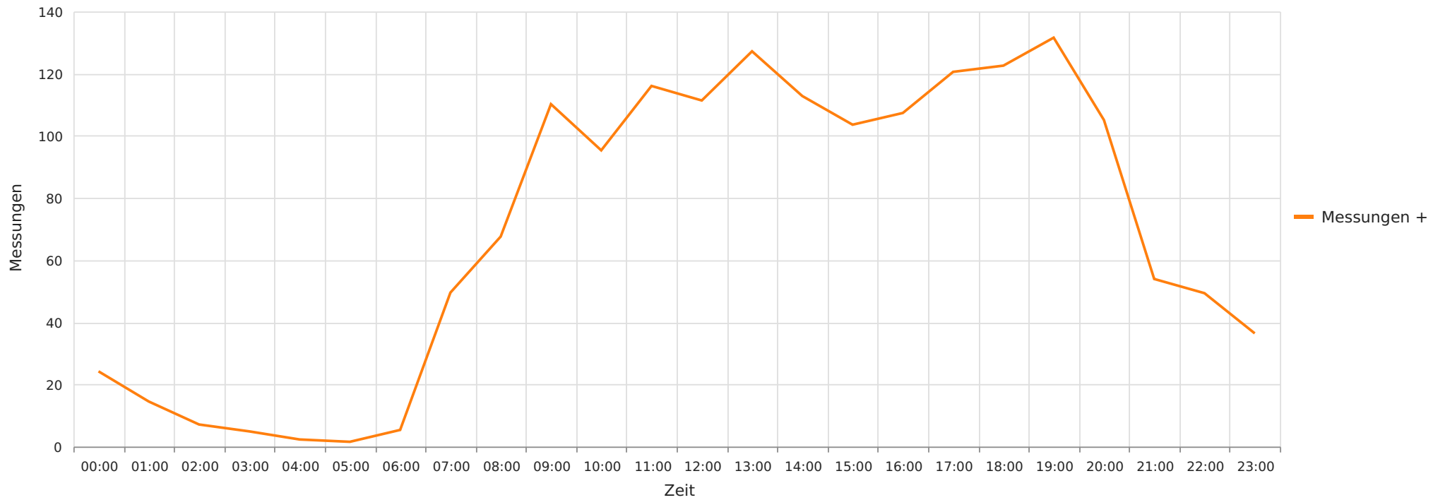
2024_03_07-04_04 Buchholz Dorfstraße Richtung B214 Gemittelte Anzahl an Messwerten vs. Uhrzeit
