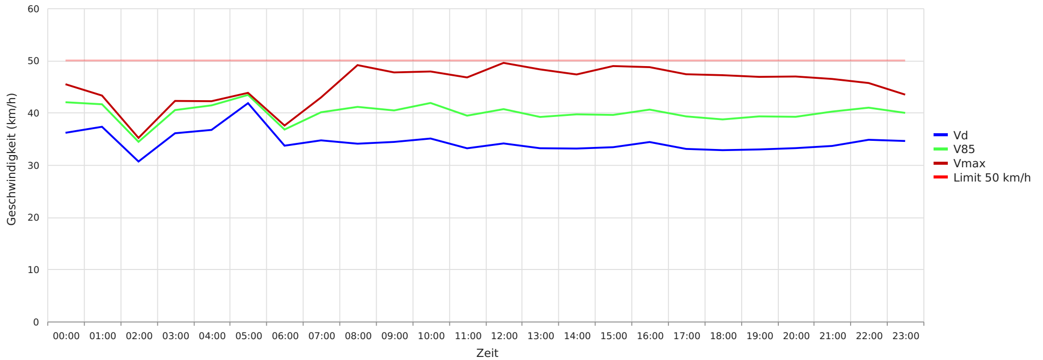
2024_03_07-04_04 Buchholz Dorfstraße Richtung B214 Vd, V85, Vmax vs. Uhrzeit
