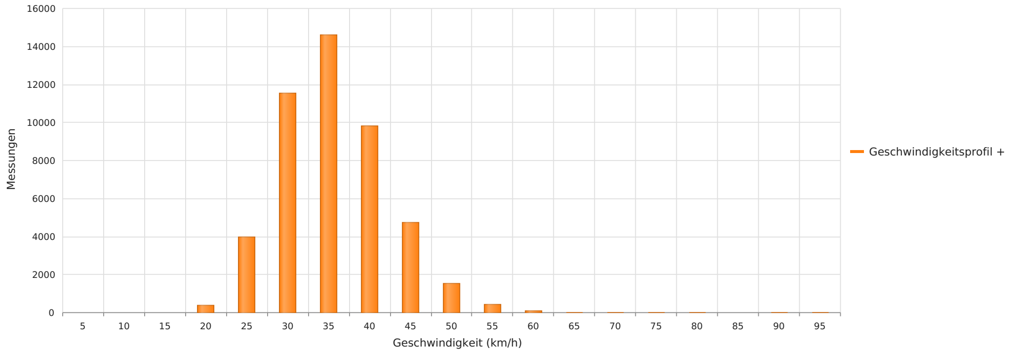
2024_03_07-04_04 Buchholz Dorfstraße Richtung B214 Anzahl der Messwerte vs. Geschwindigkeit
