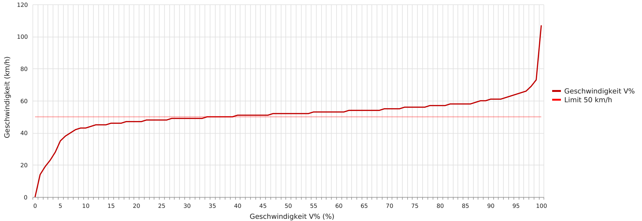
2024_08_16-09_04 Neustädter Straße Ri Ortskern Geschwindigkeit vs. prozentueller Anteil an Messwerten
