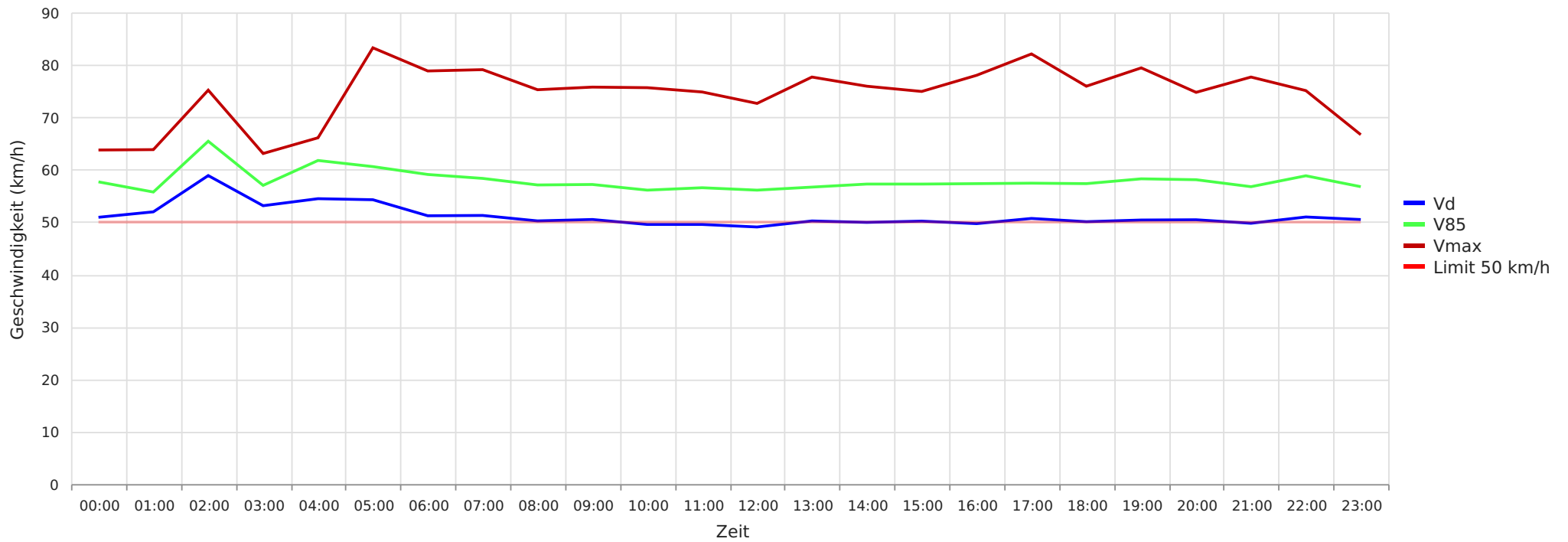
2024_08_16-09_04 Neustädter Straße Ri Ortskern Vd, V85, Vmax vs. Uhrzeit
