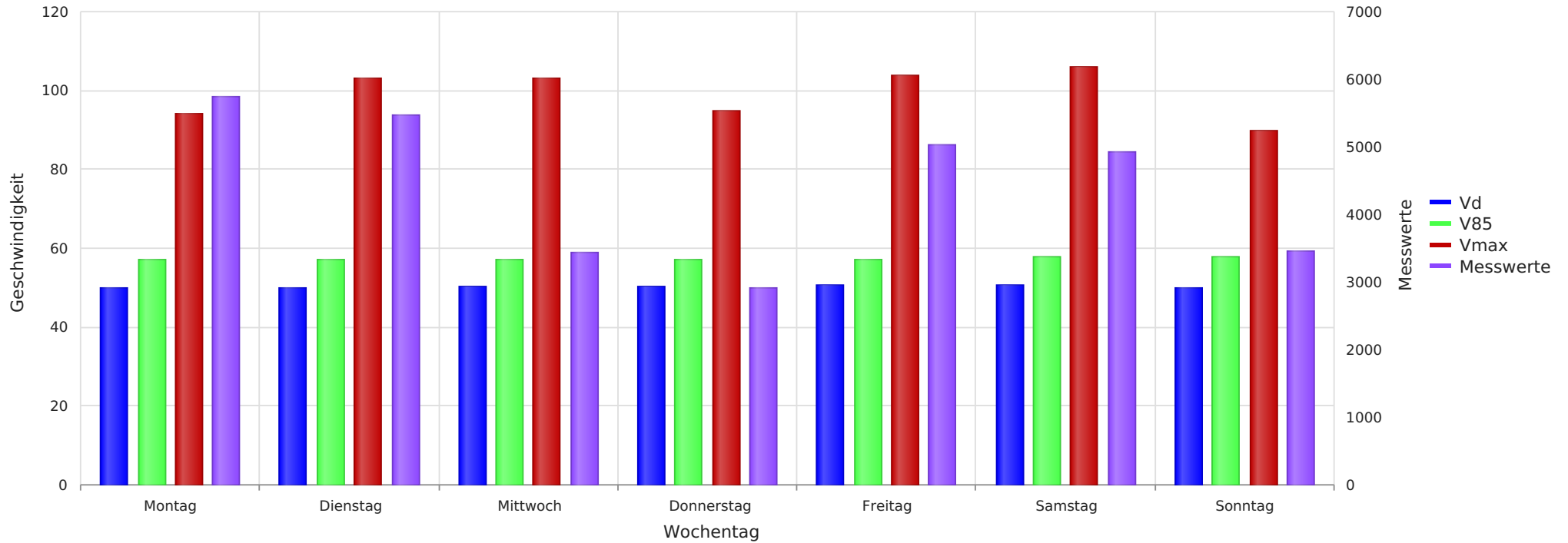
2024_08_16-09_04 Neustädter Straße Ri Ortskern Vd, V85, Vmax, Anzahl der Messwerte vs. Wochentag
