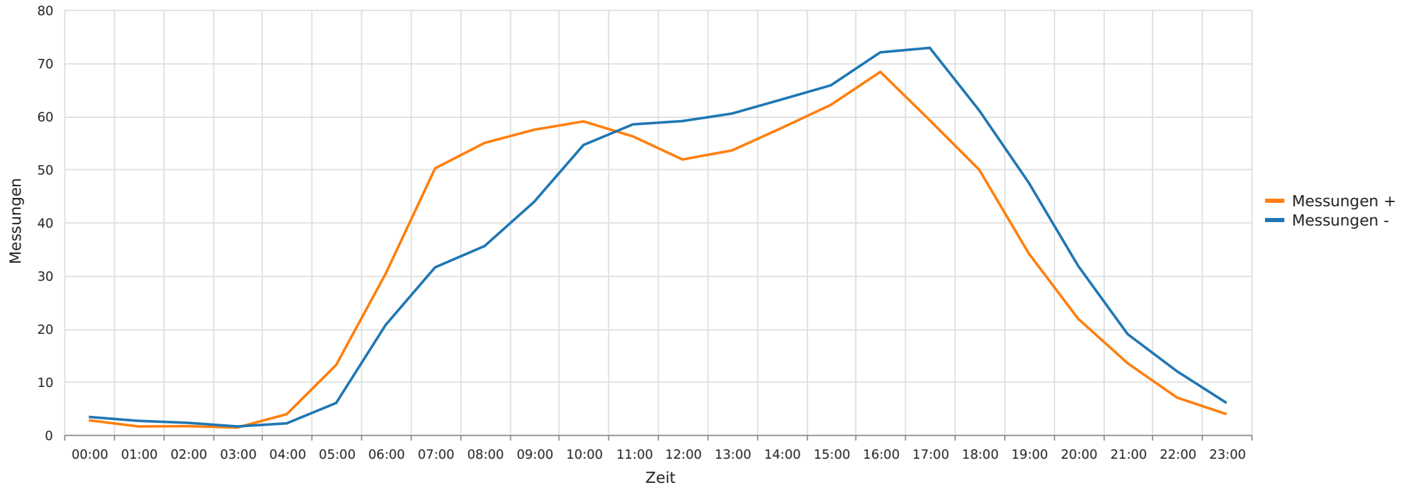
2024_08_16-09_04 Neustädter Straße Ri Ortskern Gemittelte Anzahl an Messwerten vs. Uhrzeit
