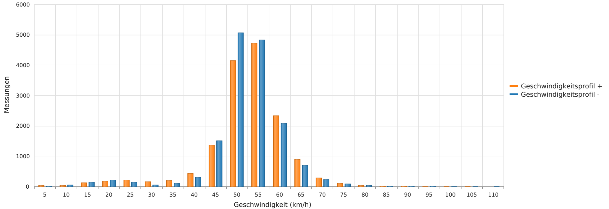
2024_08_16-09_04 Neustädter Straße Ri Ortskern Anzahl der Messwerte vs. Geschwindigkeit
