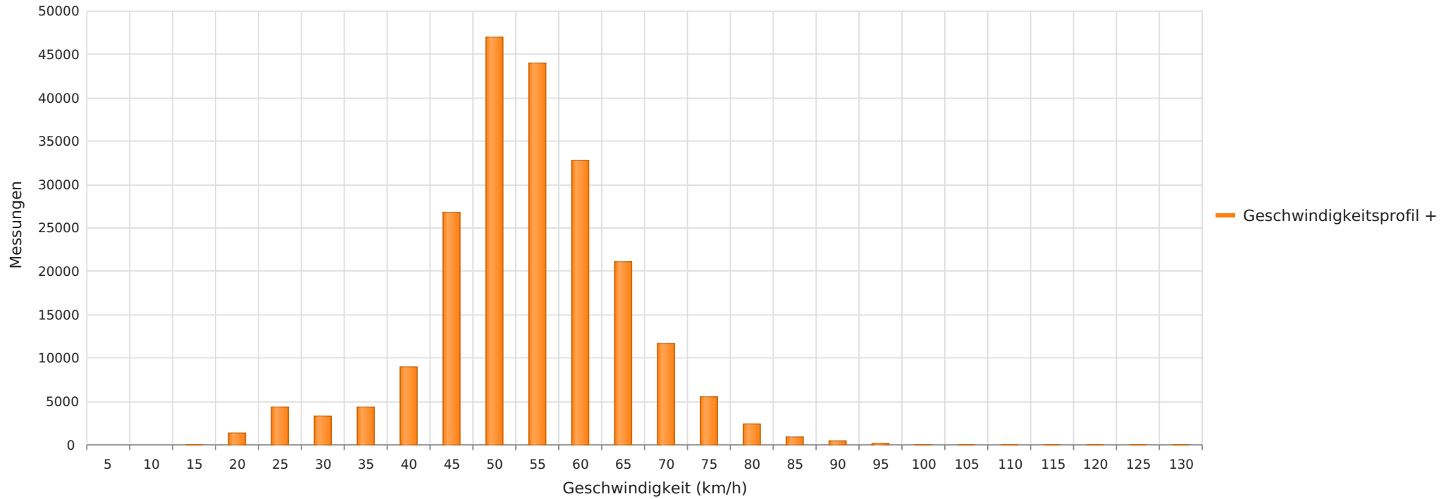
2024_08_16-2024_09_14 Essel K105 Richtung Ortskern Anzahl der Messwerte vs. Geschwindigkeit
