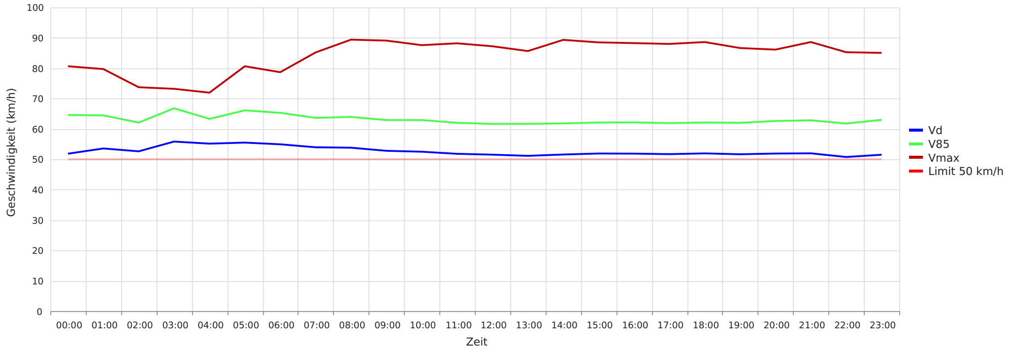
2024_08_16-2024_09_14 Essel K105 Richtung Ortskern Vd, V85, Vmax vs. Uhrzeit
