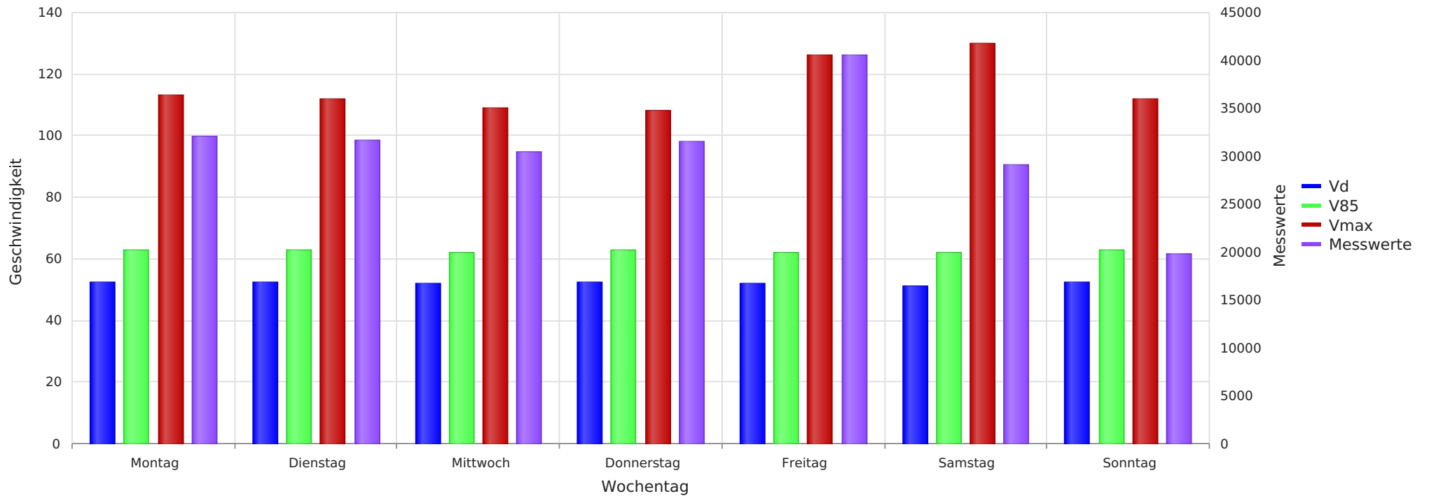
2024_08_16-2024_09_14 Essel K105 Richtung Ortskern Vd, V85, Vmax, Anzahl der Messwerte vs. Wochentag
