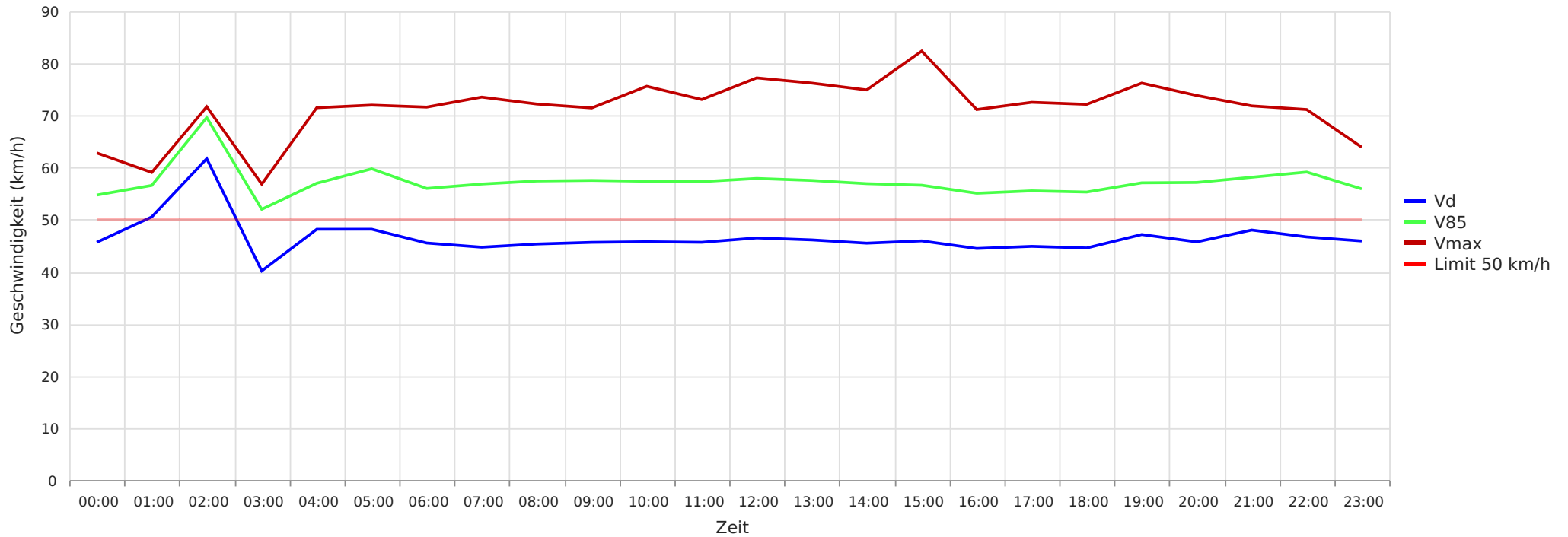
2024_11_15-2024_11_28 Hope Ortsdurchfahrt Richtung Lindwedel Vd, V85, Vmax vs. Uhrzeit
