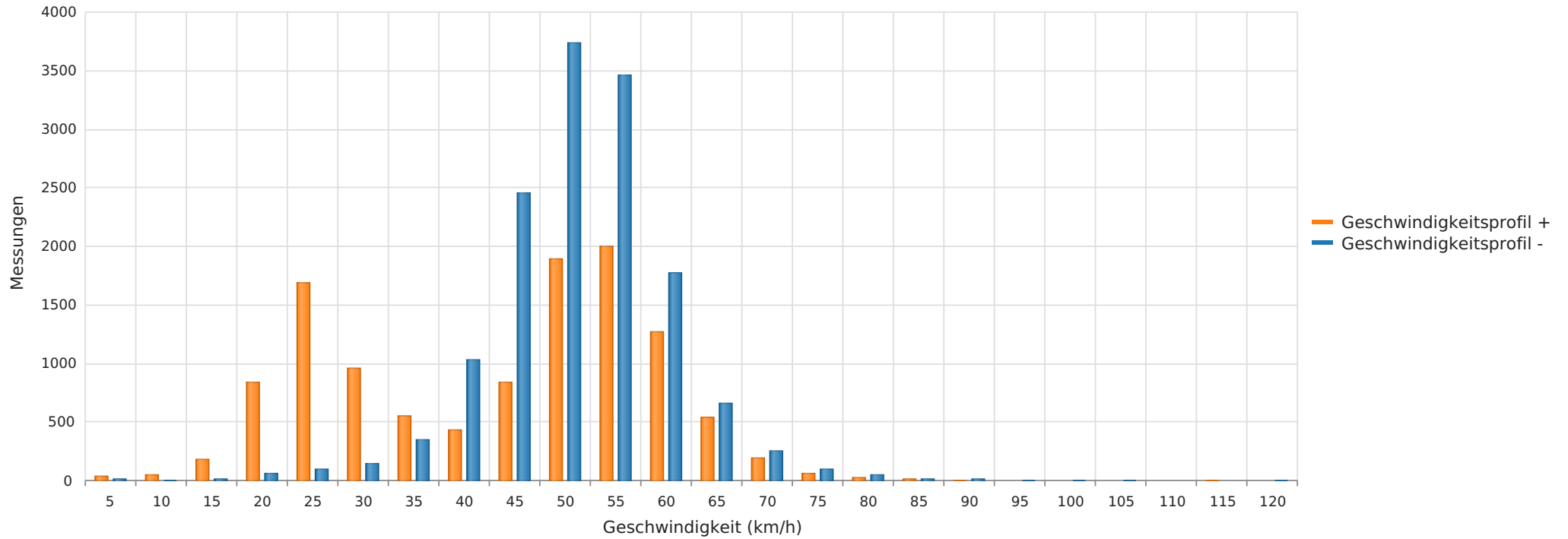
2024_11_15-2024_11_28 Hope Ortsdurchfahrt Richtung Lindwedel Anzahl der Messwerte vs. Geschwindigkeit
