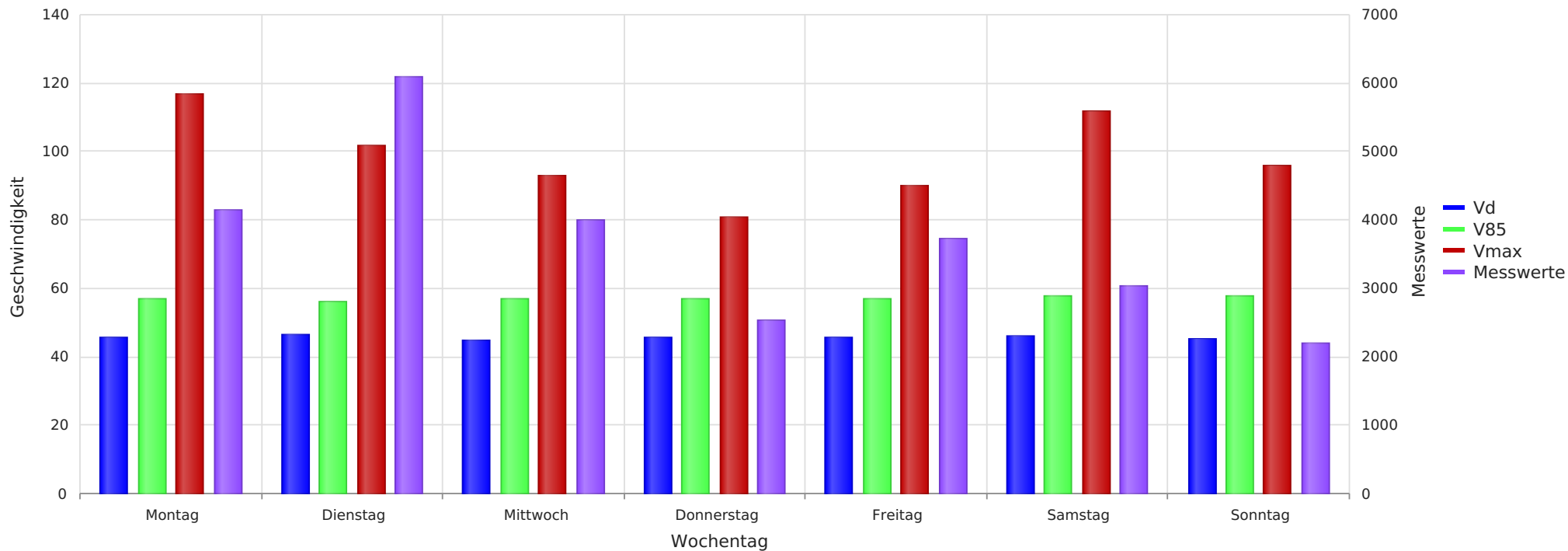
2024_11_15-2024_11_28 Hope Ortsdurchfahrt Richtung Lindwedel Vd, V85, Vmax, Anzahl der Messwerte vs. Wochentag
